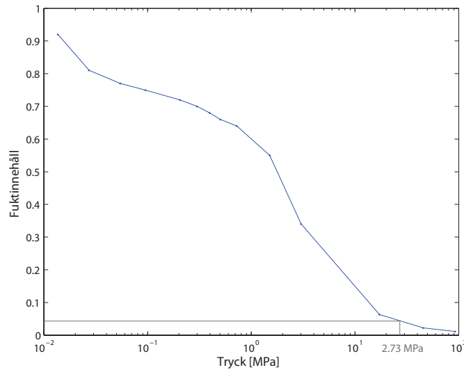
Figur 2.5 En kvalitativ illustration av fuktimhåll som funktion av porvattenundertrycket.
